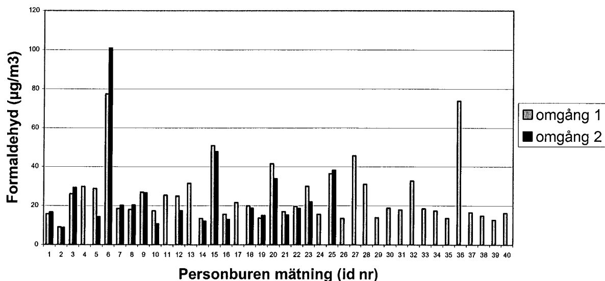
Figur 2. Formaldehydkoncentrationen ( \mu\text{g}/\text{m}^3 ) vid personburna mätningar. Upprepade mätningar utfördes på 20 personer (omgång 2).
